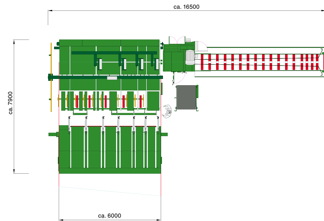
Draufsicht Manipulationsbereich, Vermessung, Einzugschisch, Besäum- und Nachschnittkreissäge DK 90 und SpreiBelabscheider
