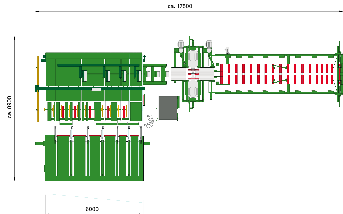
Draufsicht Manipulationsbereich, Vermessung, Einzugstisch, Besäum- und Nachschnittkreissäge BNK und Spreißelabscheider
